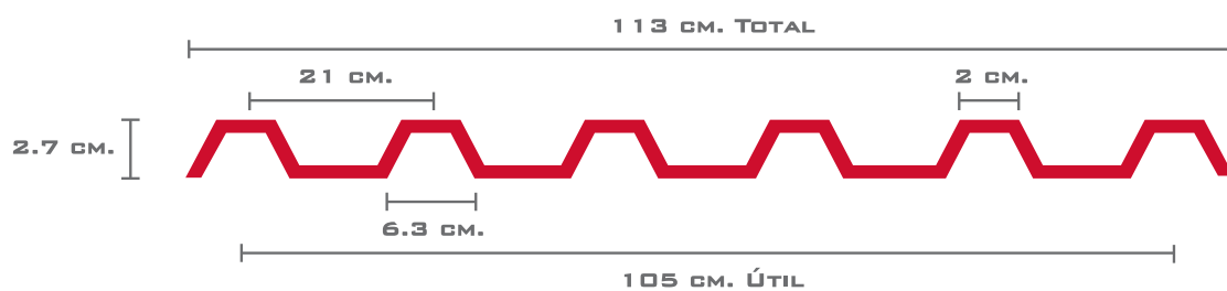
TRAPEZOIDAL OB TRASLÚCIDA
