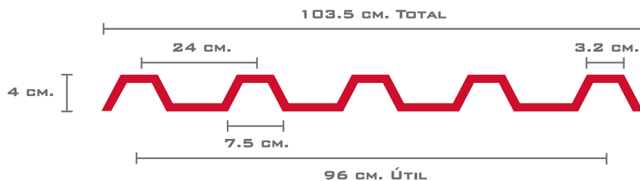
TRAPEZOIDAL OA TRASLÚCIDA
